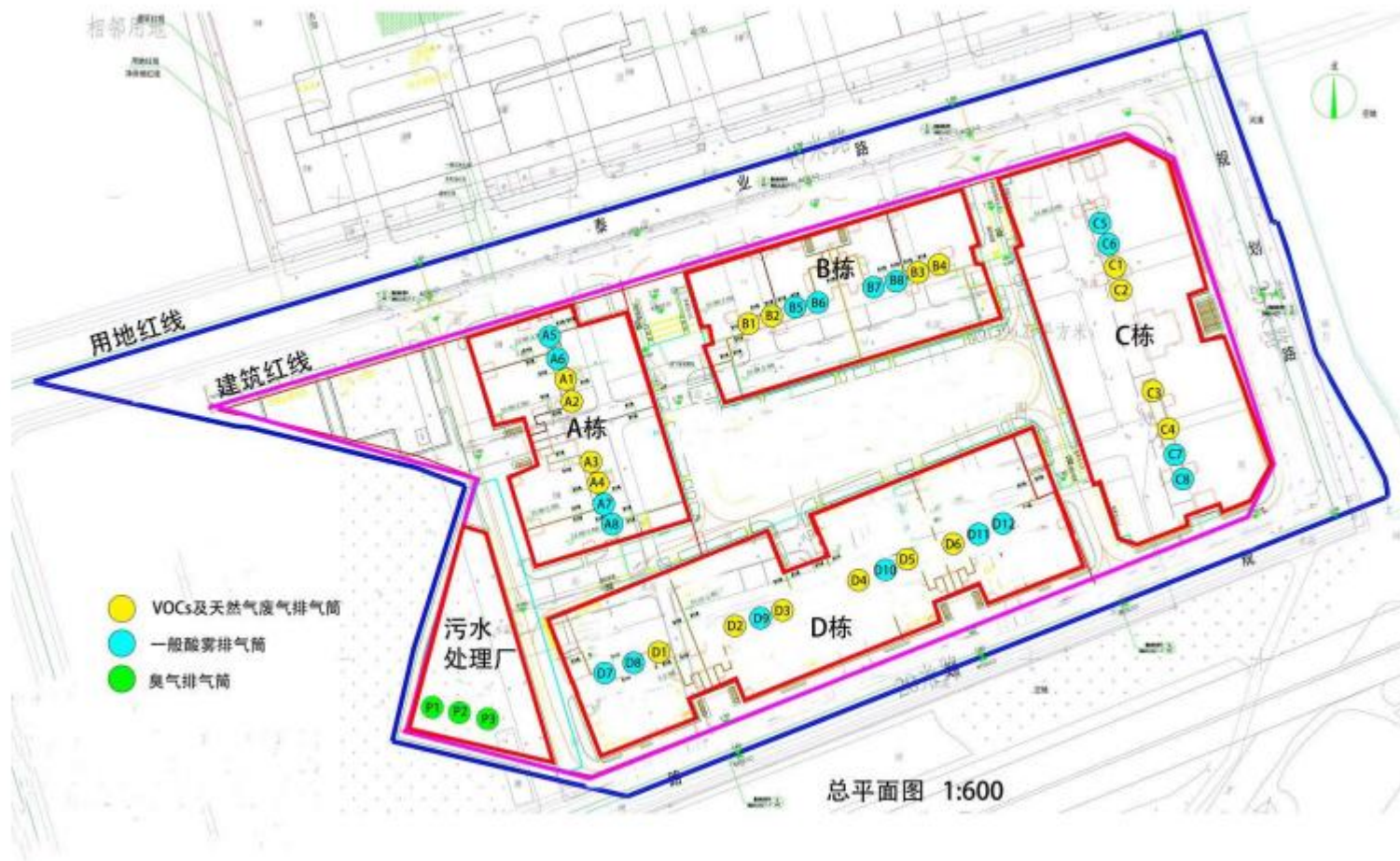
图 3.2-6 核心区平面布置图
