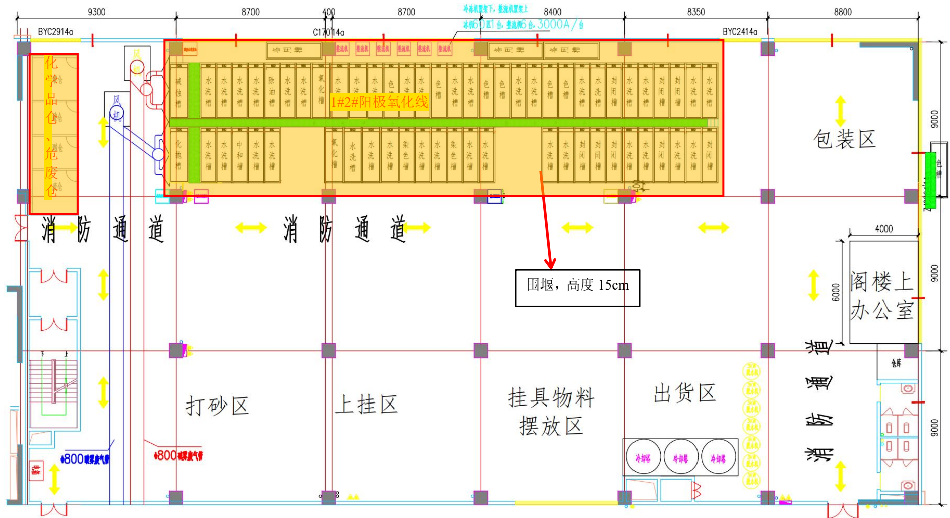
图 7.9-2 本项目防腐围堰设计图
