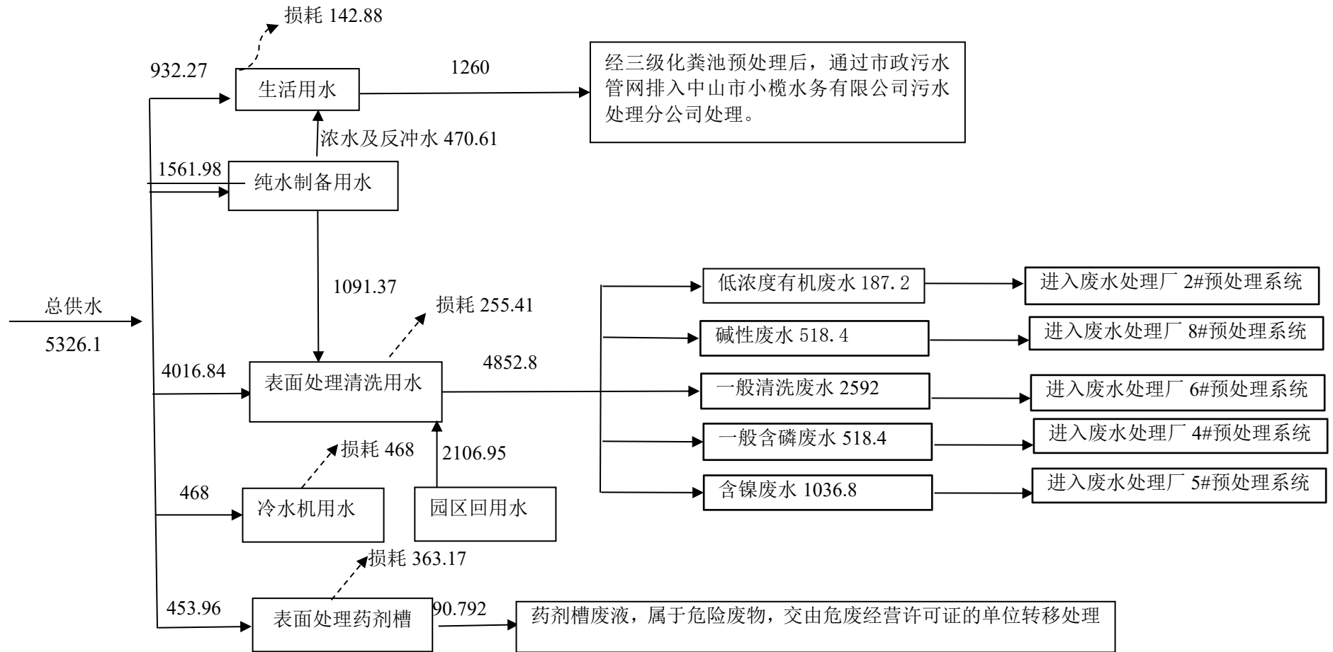
图 3.2-5 项目年水平衡图（园区提供回用水情况下） 单位： \text{m}^3/\text{a}
